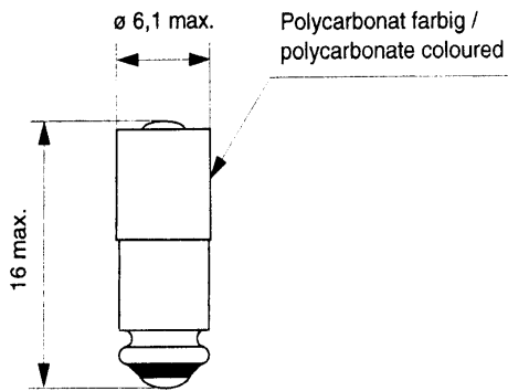
Lampensockel nach DIN EN 60061-1: S5,7s Lamp base in accordance to DIN EN 60061-1: S5,7s
