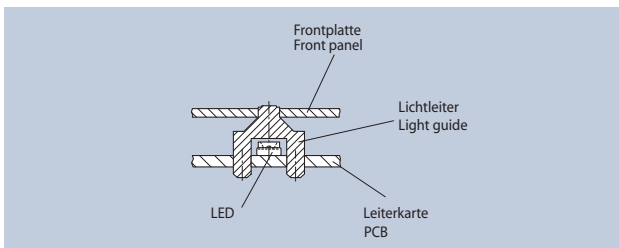
Einbaubeispiel · Mounting Example
