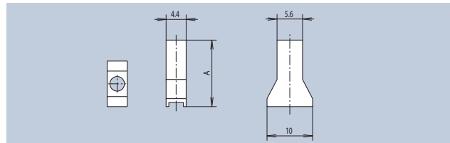
Überstrahlenschutz · Cover
