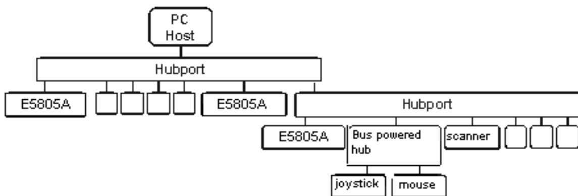
図 1 ハブのアーキテクチャ
