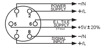
Fig. 46 Models 077-DA2, 077-DAA 077-DAB, 077-DAK, 077-DAT 077-DAV, 077-DAW LCD Digital/Analogue Meter.
