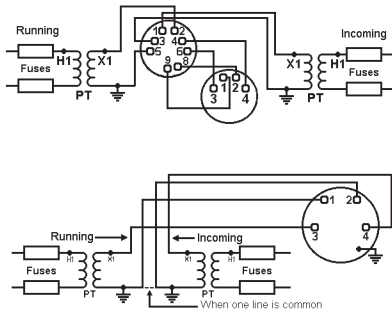
Fig. 10 Models 077-144, 077-145 077-146, 077-147, 078-144J, 078-145J 078-146J, 078-147J, 079-144, 079-145 079-146 360 Degree Dynamometer Synchroscope.
