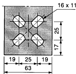
1250 A terminal lugs
