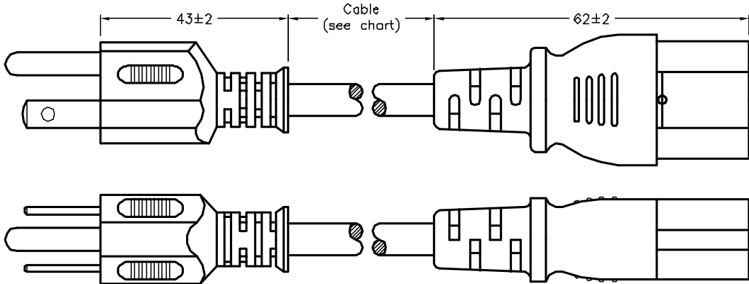
Plug NEMA 5-15P
