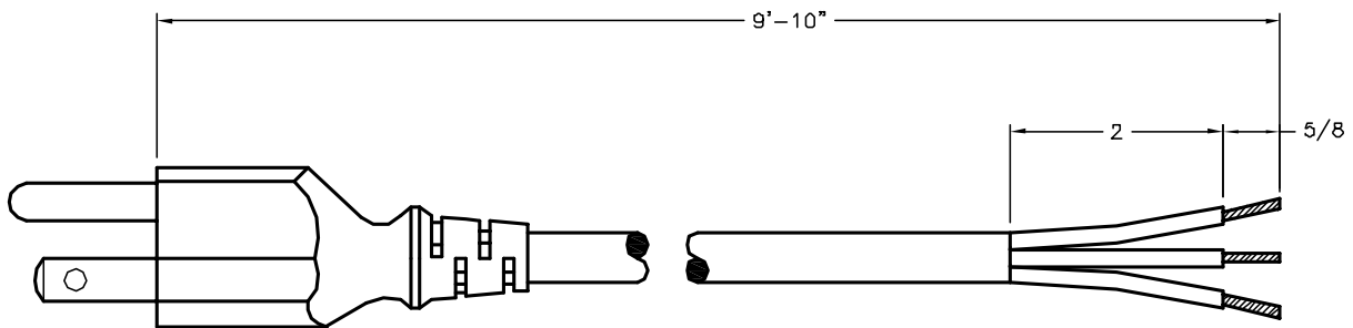
NEMA 5-15P
