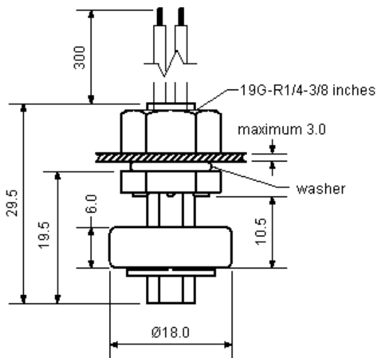
Dimensions : Millimetres
