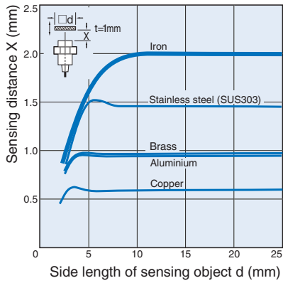
E2A-S08□N02
