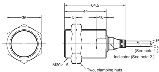
E2A-M30KS10-WP-□□/E2A-S30KS10-WP-□
