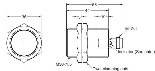
E2A-M30KS10-M1-□□/E2A-S30KS10-M1-□
