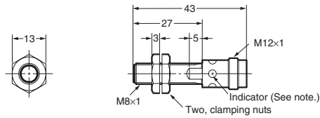
E2A-S08KS01-M1-□□
