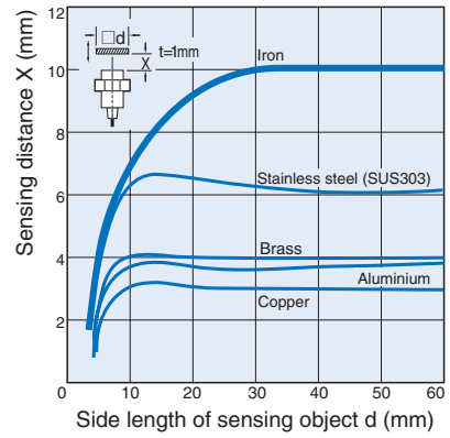
E2A-M18□N10/E2A-S18□N10
