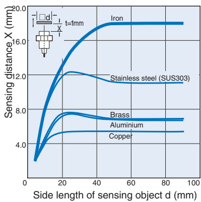
E2A-M30□N18/E2A-S30□N18
