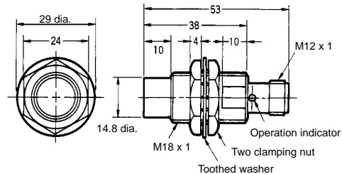
Fig. 26 : E2E-X20MD□-M1G/E2E-X18ME□-M1/F□-M1 E2E-X18MY□-M1
