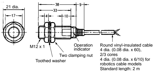
Fig. 8 : E2E-X3D□-N E2E-X2E□/F□
