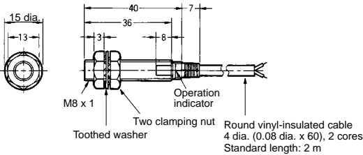
Fig. 8 : E2E-X3D□-N E2E-X2E□/F□
