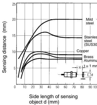
E2E-X20MD□
