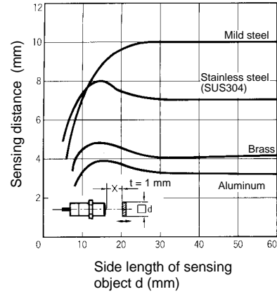
E2E-X10ME□/F□ E2E-X10MY
