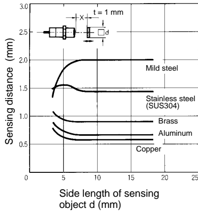
E2E-X10D□ E2E-X10T1
