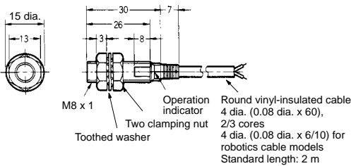
Fig. 6 : E2E-X1R5Y□
