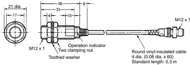
Fig. 30 : E2E-X8MD1-M1GJ
