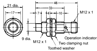
Fig. 22 : E2E-X5MY□-M1
