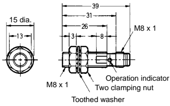
Fig. 27 : E2E-X2D□-M3G/E2E-X1R5E□-M3/F□-M3
