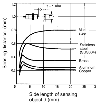
E2E-CR8□□
