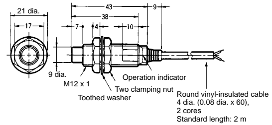
Fig. 11 : E2E-X5MY
