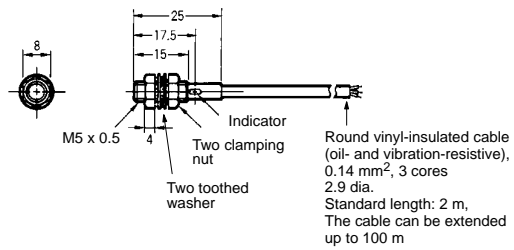
Fig. 2 : E2E-X1□□
