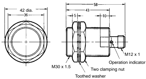
Fig. 25 : E2E-X10D□-M1G/E2E-X10E□-M1/F□-M1 E2E-X10Y1-M1
