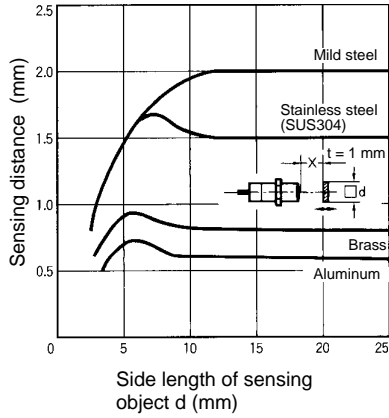
E2E-X2ME□/F□ E2E-X2MY□
