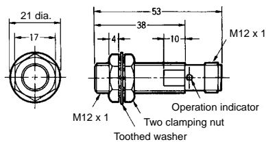
Fig. 23 : E2E-X7D□-M1G/E2E-X5E□-M1/F□-M1 E2E-X5Y1-M1
