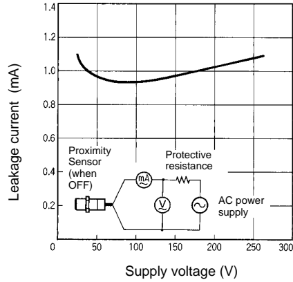
E2E-X□Y□
