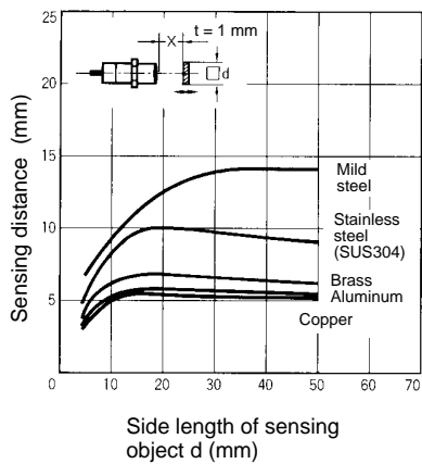
E2E-X14MD□
