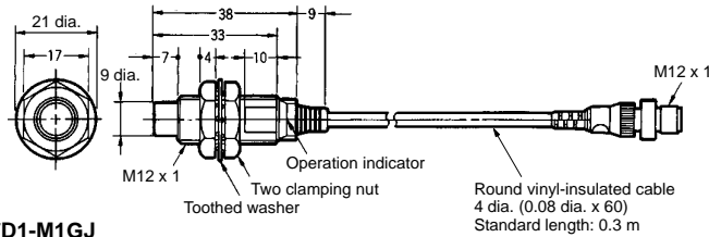
Fig. 31 : E2E-X7D1-M1GJ E2E-X7D1-M1J-T
