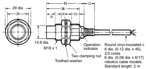
Fig. 16 : E2E-X20MD/E2E-X18ME-F E2E-X18MY
