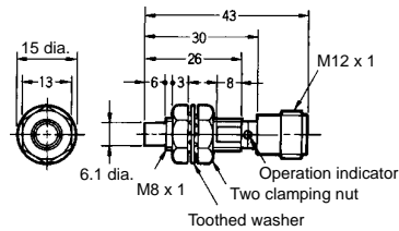
Fig. 20 : E2E-X8MD□-M1G E2E-X5ME□-M1/F□-M1
