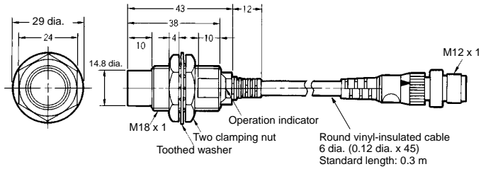
Fig. 32 : E2E-X14MD1-M1GJ
