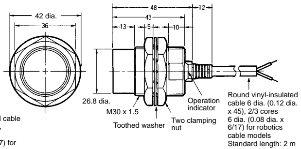
Fig. 16 : E2E-X20MD/E2E-X18ME-F E2E-X18MY
