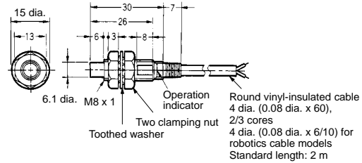
Fig. 7 : E2E-X2MY□
