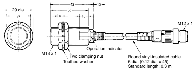
Fig. 31 : E2E-X7D1-M1GJ E2E-X7D1-M1J-T
