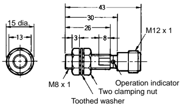
Fig. 19 : E2E-X3D□-M1G E2E-X2E□-M1/F□-M1
