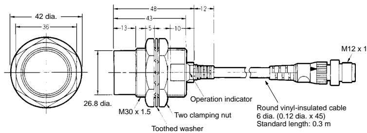
Fig. 34 : E2E-X20MD1-M1GJ
