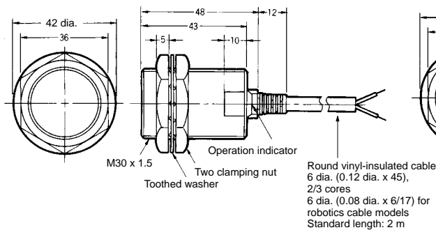
Fig. 15 : E2E-X10D-N/E2E-X10E-F E2E-X10Y/E2E-X10T1
