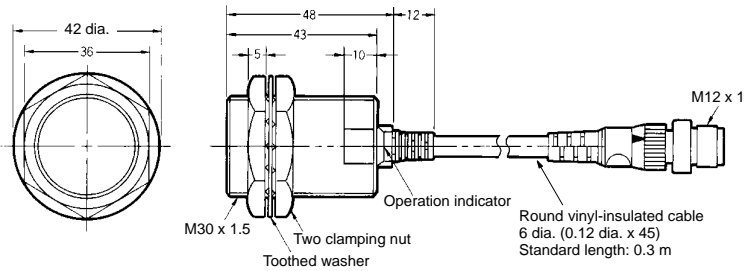
Fig. 34 : E2E-X20MD1-M1GJ
