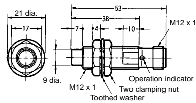
Fig. 24 : E2E-X14MD□-M1GE2E-X10ME□-M1/F□-M1 E2E-X10MY□-M1
