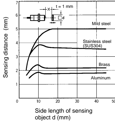
E2E-X5ME□/F□ E2E-X5MY□
