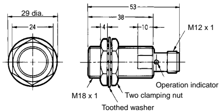
Fig. 25 : E2E-X10D□-M1G/E2E-X10E□-M1/F□-M1 E2E-X10Y1-M1
