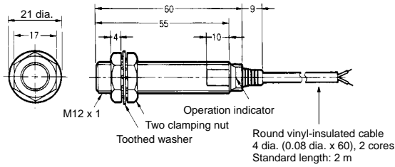
Fig. 13 : E2E-X7D-N/E2E-X5E-F E2E-X5Y/E2E-X7T1
