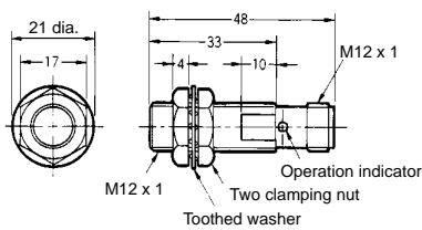
Fig. 21 : E2E-X2Y1-M1
