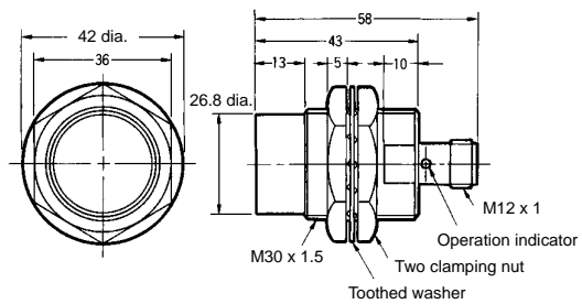
Fig. 26 : E2E-X20MD□-M1G/E2E-X18ME□-M1/F□-M1 E2E-X18MY□-M1
