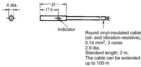
Fig. 3 : E2E-C1□□
