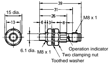
Fig. 28 : E2E-X4MD□-M3G/E2E-X2ME□-M3/F□-M3
