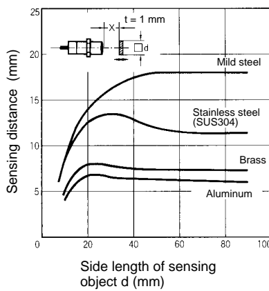
E2E-X18ME□/F□ E2E-X18MY□
