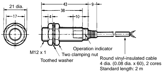
Fig. 10 : E2E-X2Y
