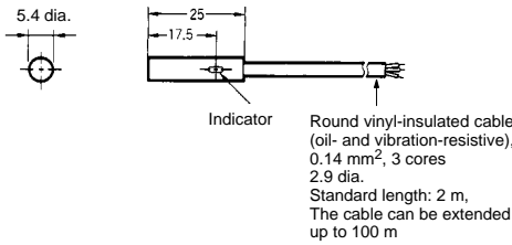
Fig. 3 : E2E-C1□□
