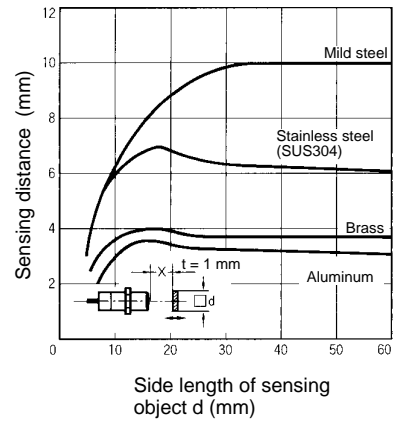
E2E-X10ME□/F□ E2E-X10MY
