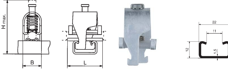
Material: Anticorodal
