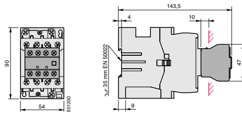
AL 26, TAL 26 + Bloque de contactos auxiliares de 4 polos frontal CA 5
