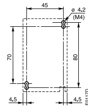
AL 30, AL 40, TAL 30, TAL 40 Plano de taladrado
