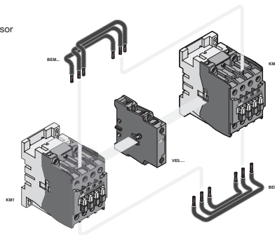
Arrancador estrella-triángulo
