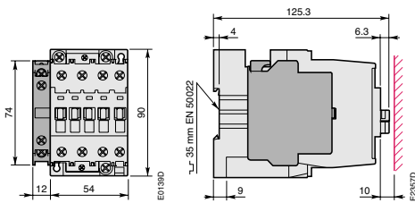
AL 30, AL 40, TAL 30, TAL 40 + Bloque de contactos auxiliares de dos polos lateral CAL 5
