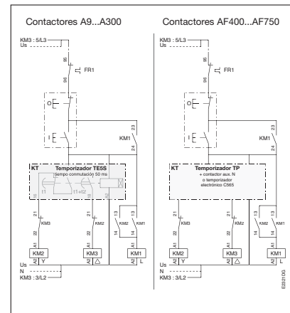
Esquema de maniobra-control remoto
