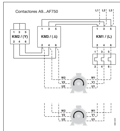
Esquema de potencia
