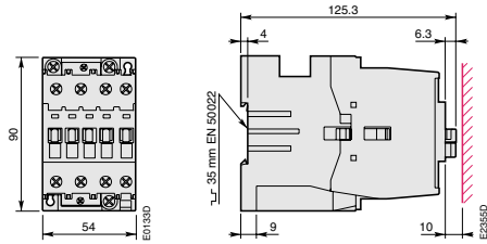
AL 30, AL 40, TAL 30, TAL 40
