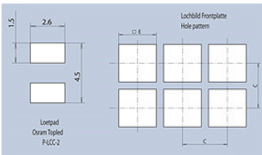
Einbaubeispiel · Mounting Example
