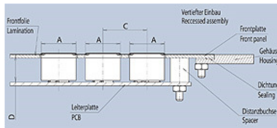
Einbaubeispiel · Mounting Example
