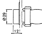
XB2-BA●● ZB2-BA●(1)
