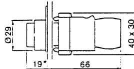
XB2-BW3●, 7● ZB2-BW1●, BW3●, ZB2-BK●●●(1) ZB2-BW07●(2)
