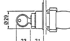
XB2-BG21 ZB2-BG●(1)
