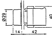
XB2-BV7● ZB2-BV0●(1) ZB2-BV7 (2)
