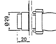
XB2-BL●● ZB2-BL●(1)
