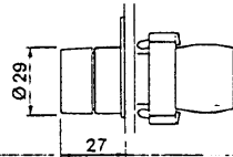
XB2-BD●● ZB2-BD●(1)
