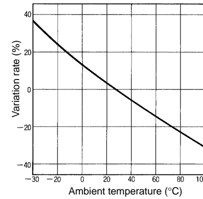
G3NA-2□□B AC Input
