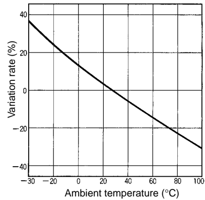
G3NA-2□□B AC Input
