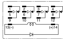
4PDT (RY4)
