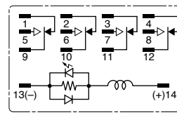
4PDT (RY4)
