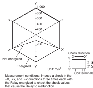
Malfunctioning Shock G6D-1A-ASI
