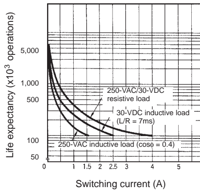
G2R-24, G2R-2A4
