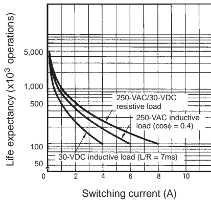
G2R-14, G2R-1A4
