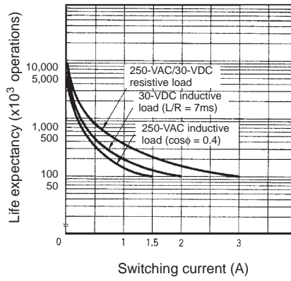
G2RK-2A, G2RK-2
