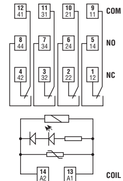
Example: AC
