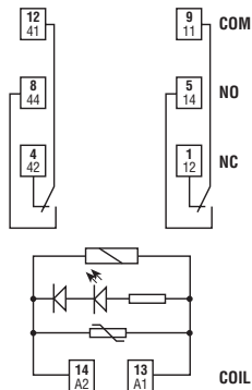
Example: AC
