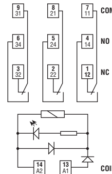
Example: DC
