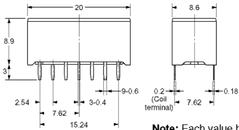
G6ZK-1P-A
