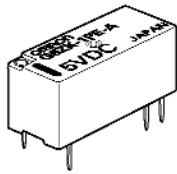
G6ZK-1PE-A
