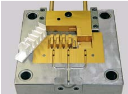
Injection moulding die
