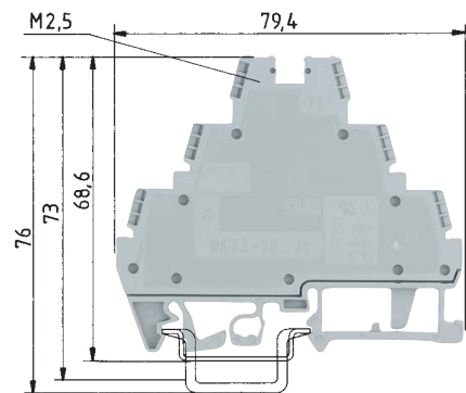
WK 2,5 - 3 D/U-NGN
