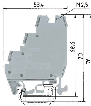
WK 2,5 - 4 KI/U-NGN
