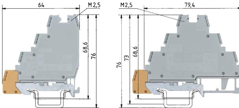
WK 2.5 - 4 KI SL-PGN WK 2.5 - 4 KI SL-PRT
