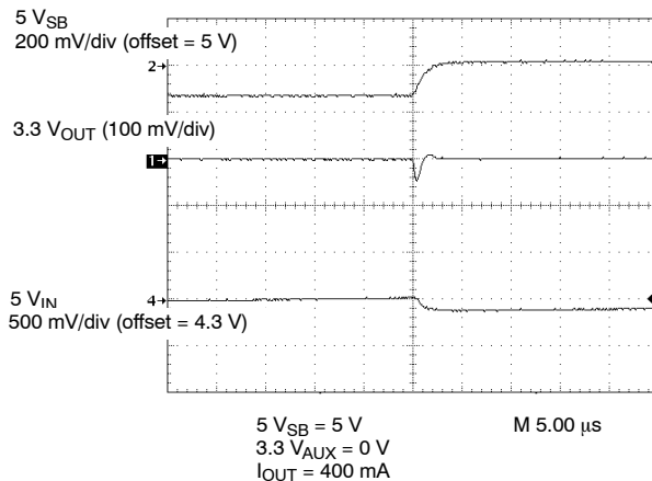
5 VIN Power Up ( 5 V_{SB} = 5 \text{ V} )
