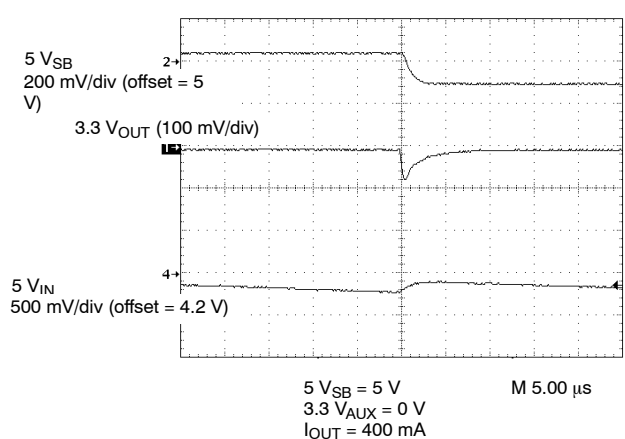
5 VIN Power Down ( 5 V_{SB} = 5 \text{ V} )
