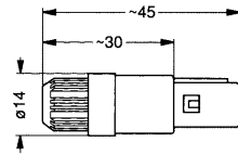
PA ● Straight plug with cable collet and nut for fitting a bend relief Gerader Stecker mit Zugentlastung und Mutter für eine Knickschutztüle
