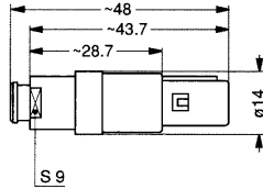
PA ● Straight plug with cable collet and nut for fitting a bend relief Gerader Stecker mit Zugentlastung und Mutter für eine Knickschutztüle
