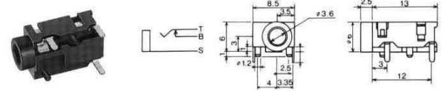
No.M03-663A0 (φ 3.5) STEREO
