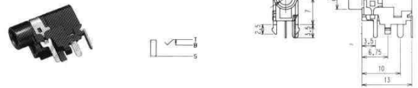
No.M03-772A0 (φ 3.5) STEREO
