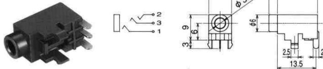
No.MX-345GLB (φ 3.5) STEREO Net Weight : 1 gr.
