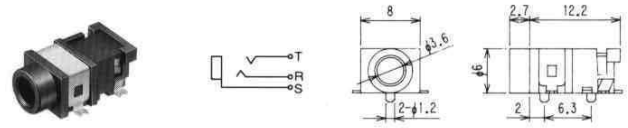
No.M03-772A0 (φ 3.5) STEREO
