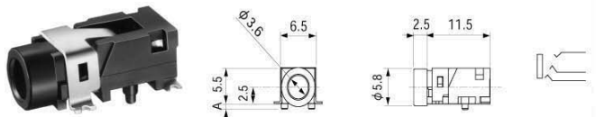
No.M03-663A0 (φ 3.5) STEREO
