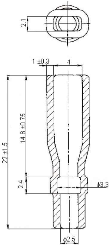
Dimensions : Millimetres
