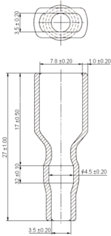
Dimensions : Millimetres
