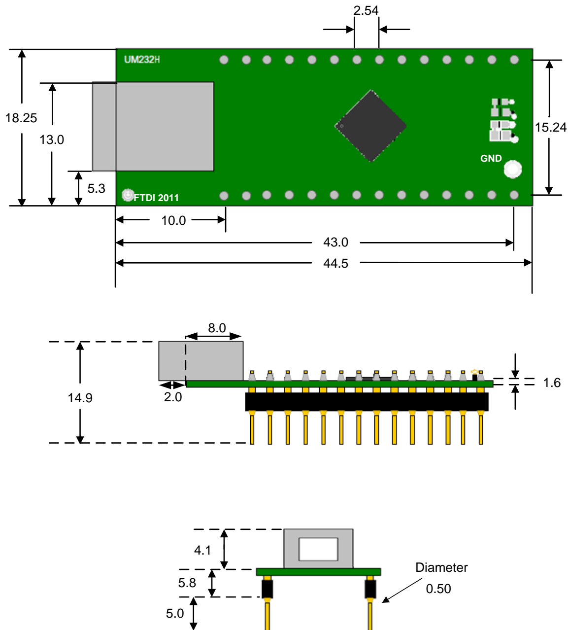
Figure 5.1 : UM232H Module Dimensions
