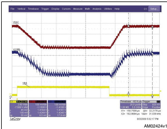
Figure 27. GFX supply - VID step, skip mode
