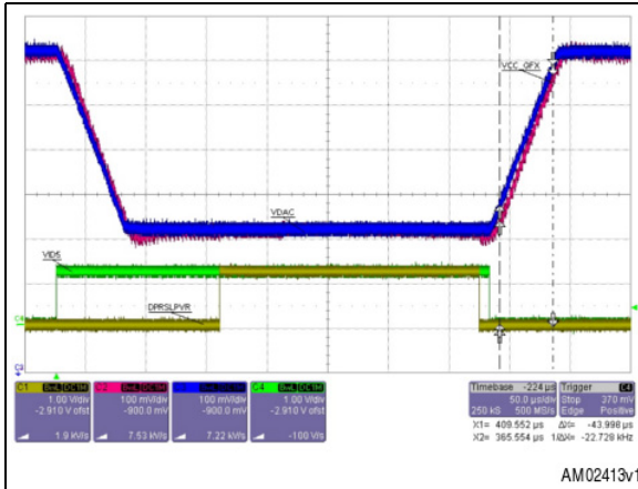
Figure 18. V CORE VID step variation - VR11 mode
