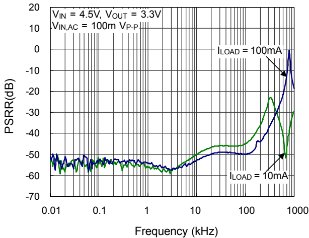
PSRR
