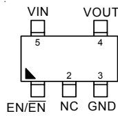
TSOT-23-5/SOT-23-5/ SC-70-5
