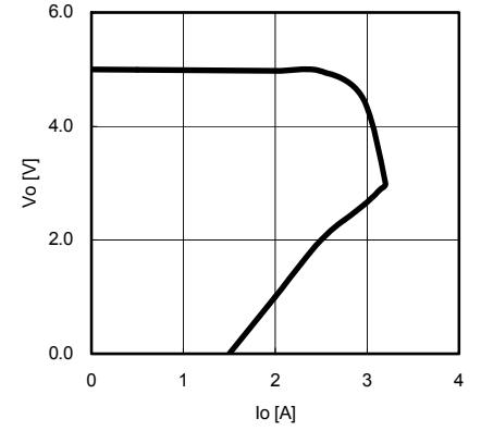
Fig. 15 OCP
