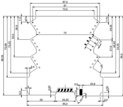
Maßbild der Leiterplatte ME MAX 3-3 für Printklemmenanschluss (MKDSO), Ansicht: Bestückungsseite
