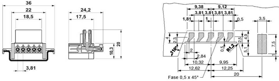
Detailmaßbild der Tragschienen- Busverbinder-Kontaktpads
