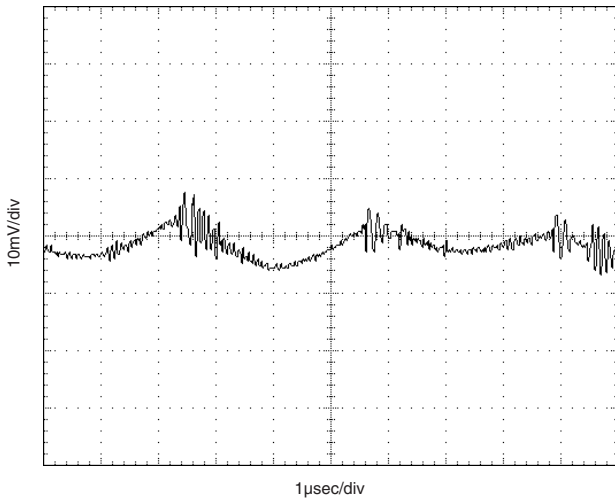
Output Ripple/Noise
