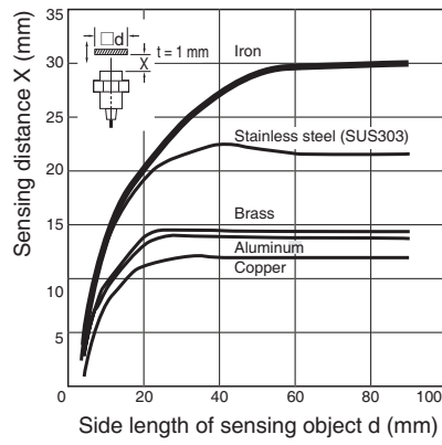
E2A-M30LN30/E2A-S30LN30
