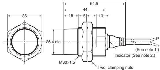
E2A-M30KN20-WP-□□/ E2A-S30KN20-WP-□
