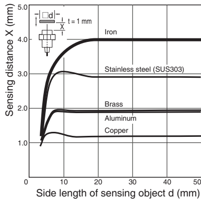
E2A-S08□N04
