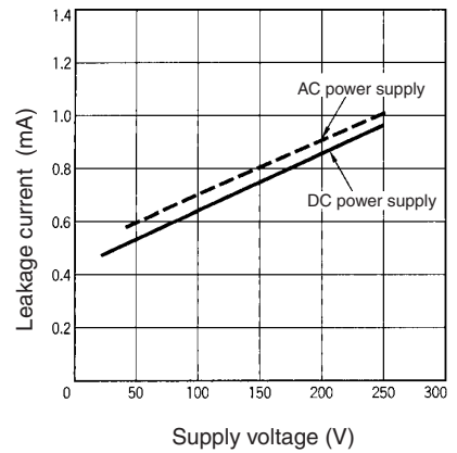
E2E-X□T1 DC/AC
