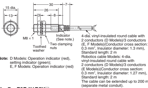
Fig. 7: E2E-X1R5Y
