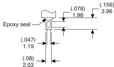
Solder Lug
