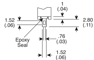
SOLDER LUG
