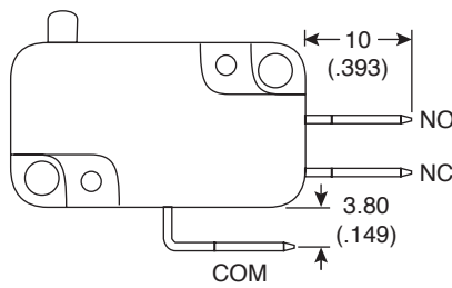
Quick connect terminal 187 series (D)
