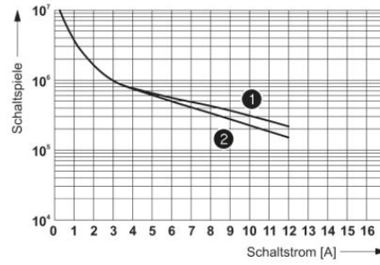
Elektrische Lebensdauer
