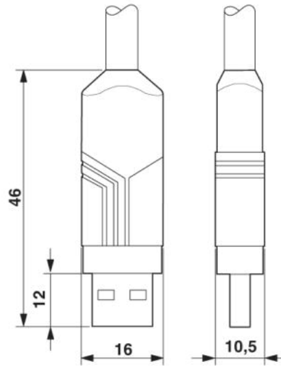
USB-Steckverbinder, Typ A, Standard
