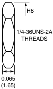
NUT
