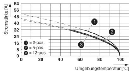
Deratingkurve für: SPC 5/...-ST-7,62 mit PC 5/...-G-7,62 Leiterquerschnitt: 6 mm 2
