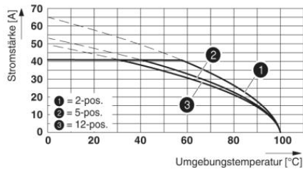
Deratingkurve für: SPC 5/...-ST-7,62 mit PC 5/...-G-7,62
