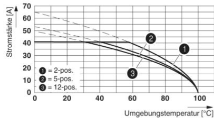
Deratingkurve für: SPC 5/...-ST-7,62 mit PC 5/...-G-7,62
