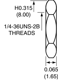
NUT
