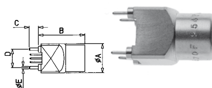
EZ : PCB
