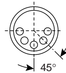
5 Pin 180° Arc 174-2512
